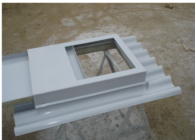
Ouverture de 50cm par 60cm de large
